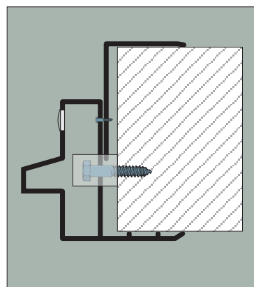
3. ID3 aluminium Foder 130-170 mm
