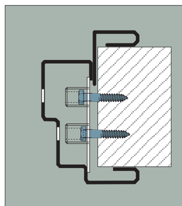
6. R3 rostfri ställbar Valfri väggjocklek
