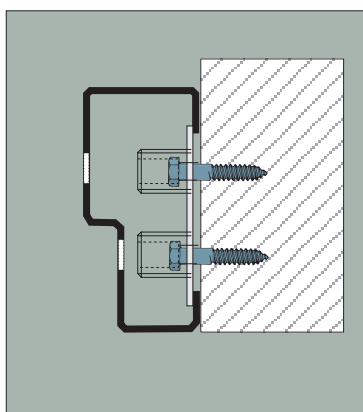
5. R2 rostfri smyg Karndjup 95 mm
